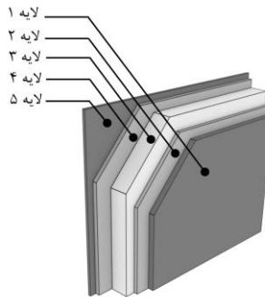
شکل ۱۹-۵-۱: نحوه محاسبه مقاومت حرارتی پوسته خارجی غیرنورگذر چند لایه
